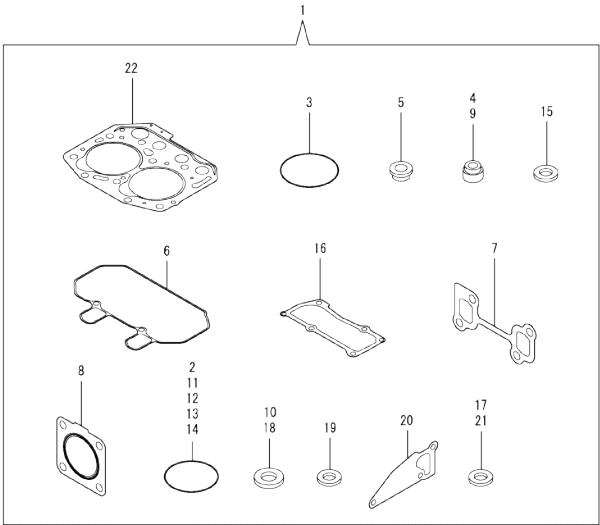
Fig.16. GASKET SET
